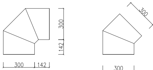
KOLENO (45°,90°)
