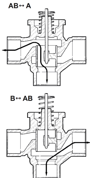
Obr. 2. Prietok kvapaliny cez 3-cestný ventil
