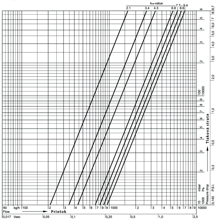
Obr. 7. Charakteristika tlakovej straty ventilu.
