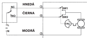
Obr. 3. Pripojenie s 3-vodičovým prevedením pomocou prepínacieho SPDT kontaktu
