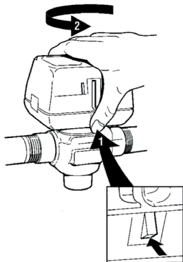
Obr. 6. Západkový mechanizmus.
