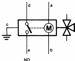
Obr. 7. Schéma zapojení ventilu.
